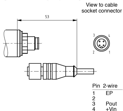
Fig. 15 - M12 x 1, 4 pins (Lumberg RSF4)
