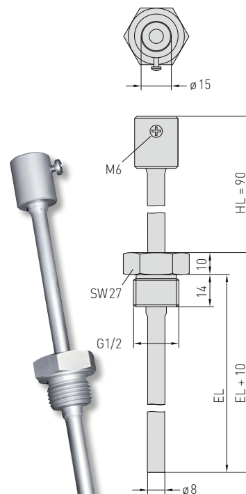
Afmetingen TH08-VA / xx / 90
