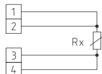
1x Четырёхпроводное подключение (опционально)
